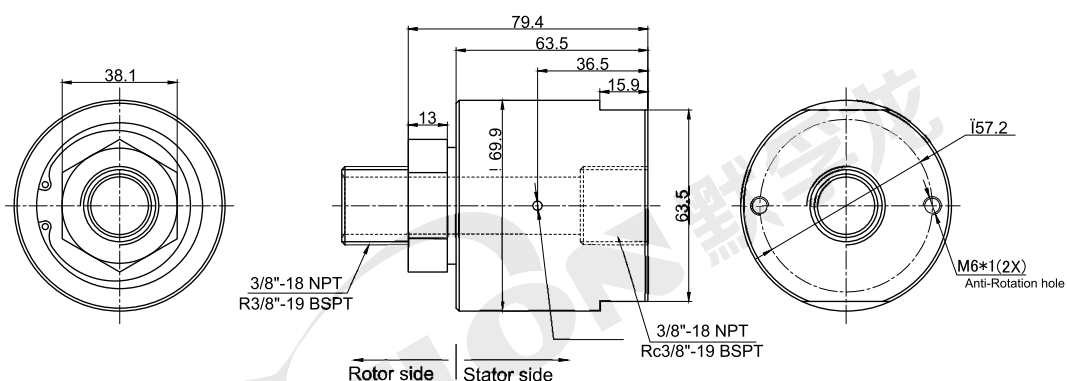
MSPS18 (单路旋转接头) 尺寸图 G1"牙
