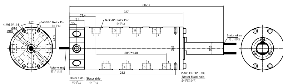
MK83S-S56 尺寸图 8进8出G3/8"牙
